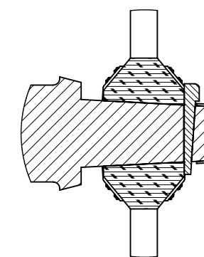
SECCIÓN B-B ESCALA 1 : 10
