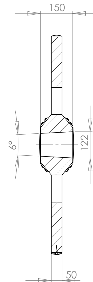
SECCIÓN A-A
